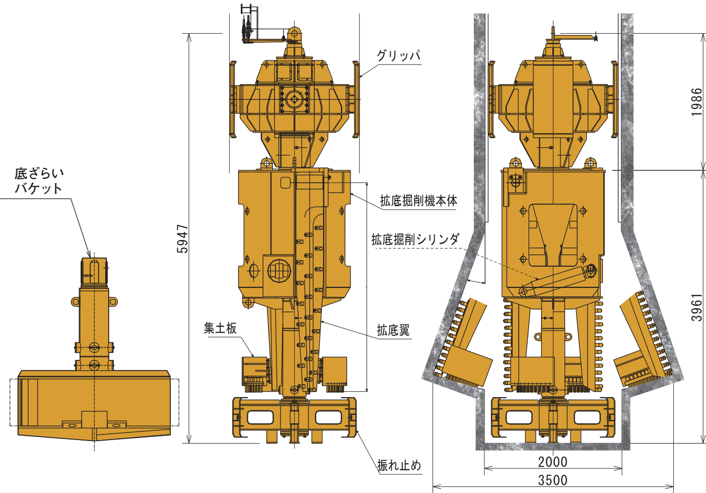
E・Rock ビット 1835 型
